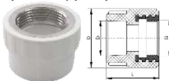
Рисунок 19. Муфта, комбинированная с внутренней резьбой
